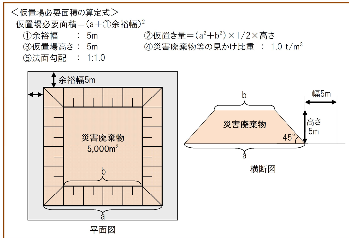
図 15 仮置場面積の模式図
