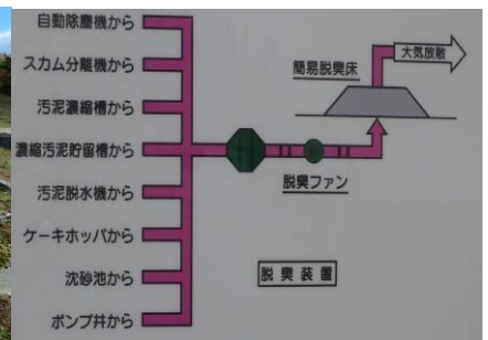
南富良野町浄化センター屋外脱臭装置
